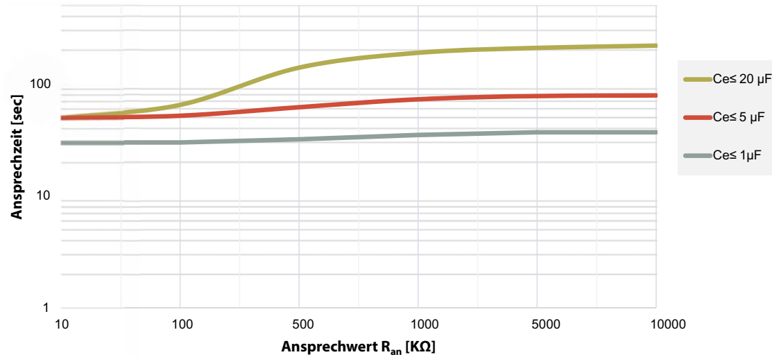
Ansprechzeit in Abhängigkeit vom Ansprechwert und Netzableitkapazität nach IEC 61557-8 ( U_n = AC\ 690\ V , f_n = 60\ Hz )
